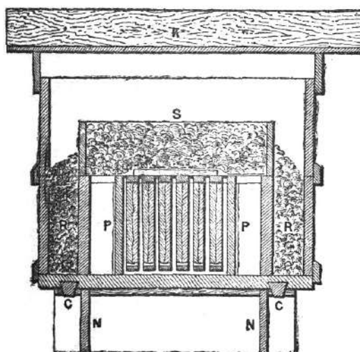
Fig. 15. Corte longitudinal de la colmena Cowan con bastidor de secciones.
