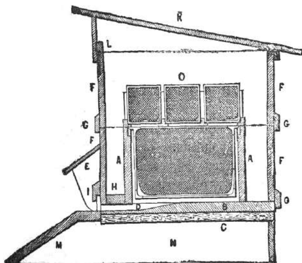
Fig. 14. Corte longitudinal de la colmena Cowan con bastidor de secciones.
