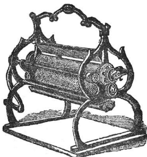
Fig. 32: Máquina Dunham.
