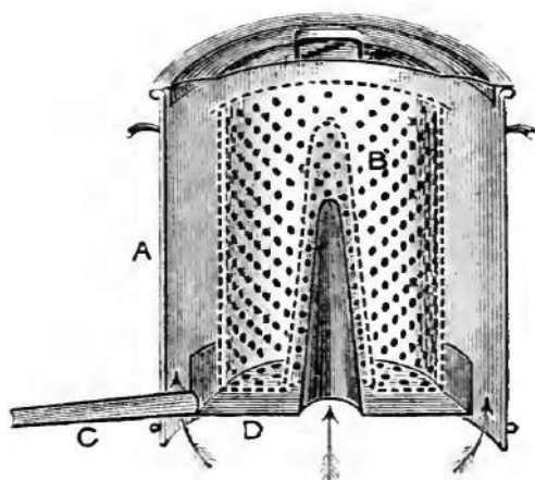
Fig. 52. Extractor de cera del profesor Gerster.
