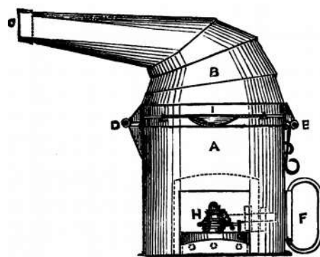
Fig. 71 bis. Fumigador Bertrand.
