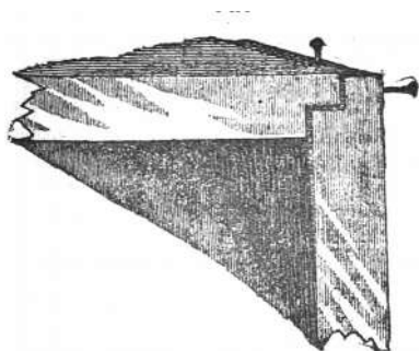
Fig. 10. Ensambladura con doble encaje.
