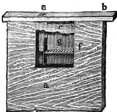
Fig. 61. Alimentador en el tabique de separación.
