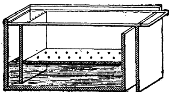
Fig. 64. Alimentador para contener \frac{1}{2} galón de jarabe.
