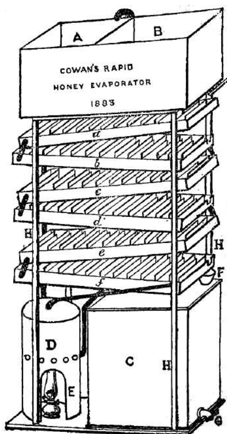
Fig. 51. Evaporador de miel.
